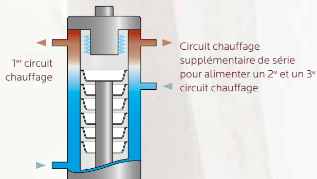
Coupe corps de chauffe Optimal avec brûleur cylindrique FLATFIRE®
