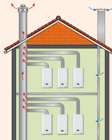
Alvéoles techniques Possibilité de poser jusqu'à 3 chaudières TRADITION Visio par alvéole
