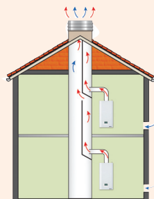
Conduit Shunt ou Alsace Voir DTU 24.1 P2
