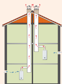
Conduit individuel À TIRAGE NATUREL B13 - BS
